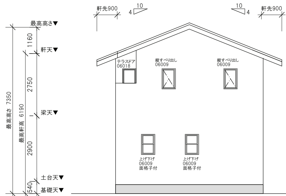
東 立面図
