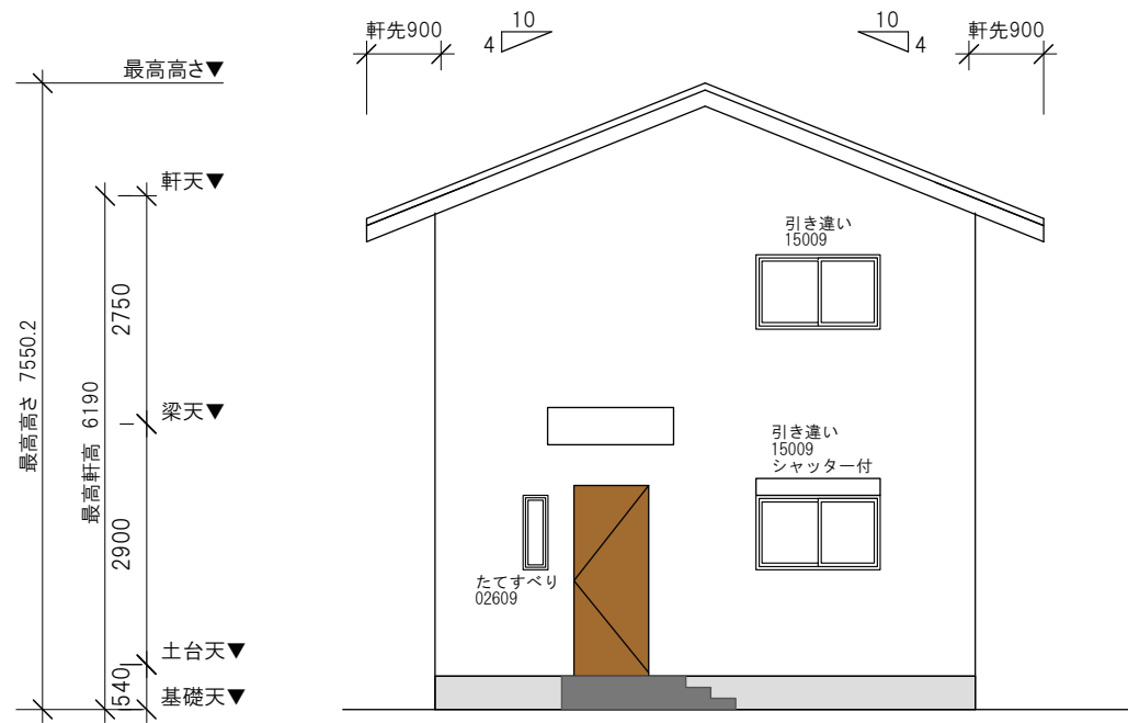
西 立面図
