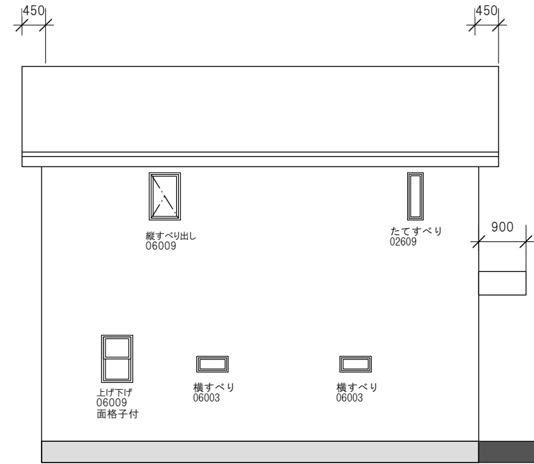
北 立面図
